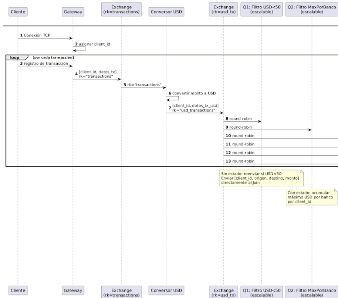
Figura 8: Primera parte del diagrama de secuencia para la ingesta de datos.
